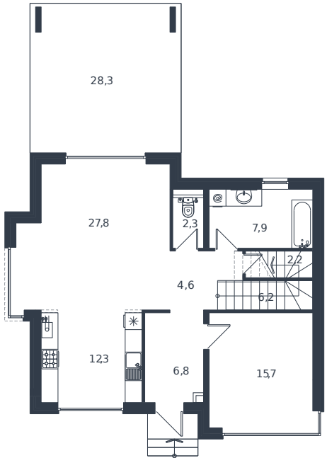
1 этаж
