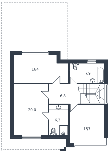
2 этаж
