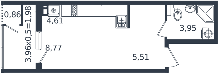
1 этаж
