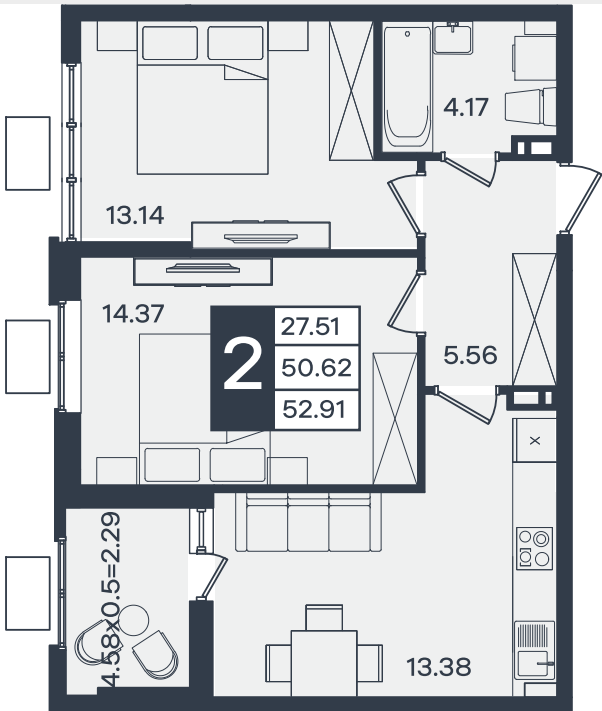
1 этаж
