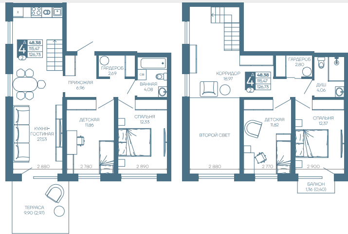
1 этаж
