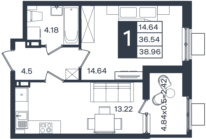
1 этаж
