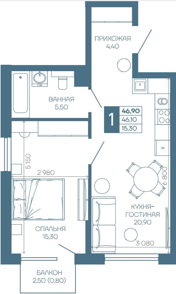
1 этаж
