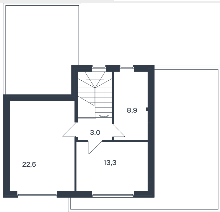
1 этаж
