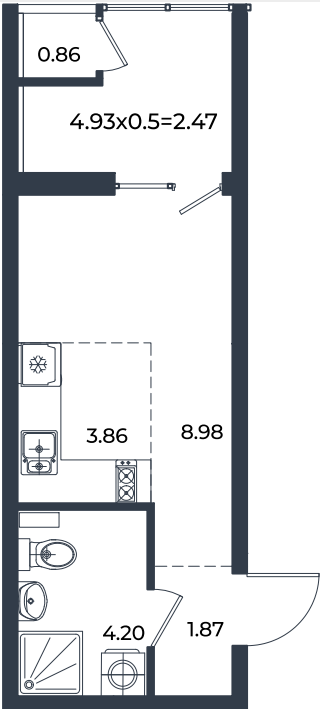
1 этаж
