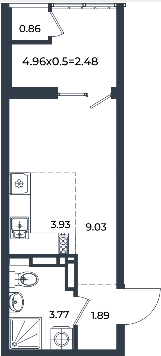
1 этаж
