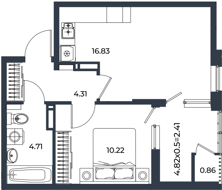
1 этаж
