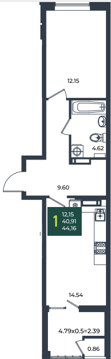
1 этаж
