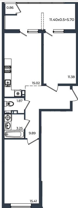
1 этаж
