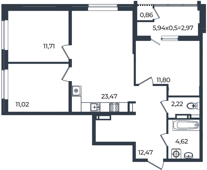
1 этаж
