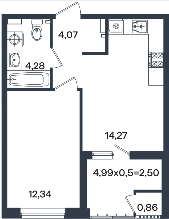
1 этаж
