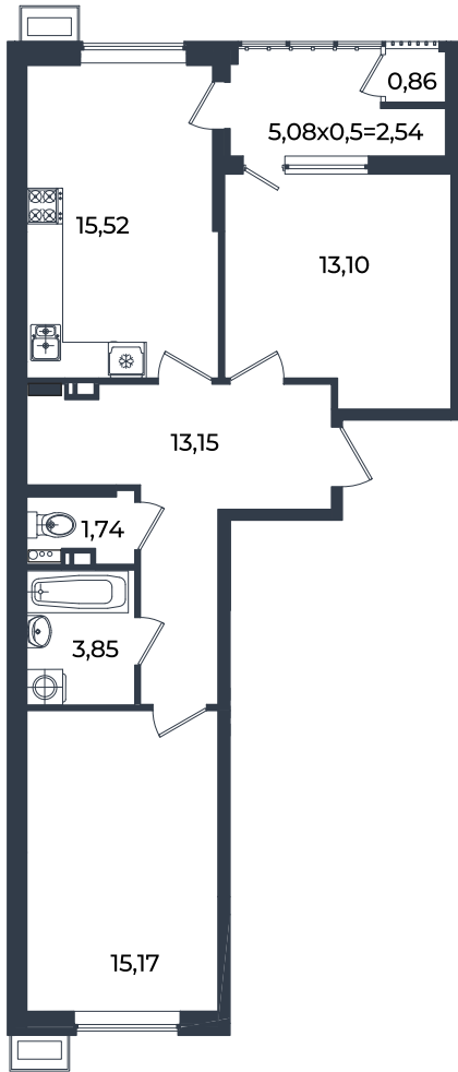
1 этаж
