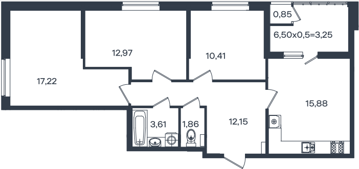
1 этаж
