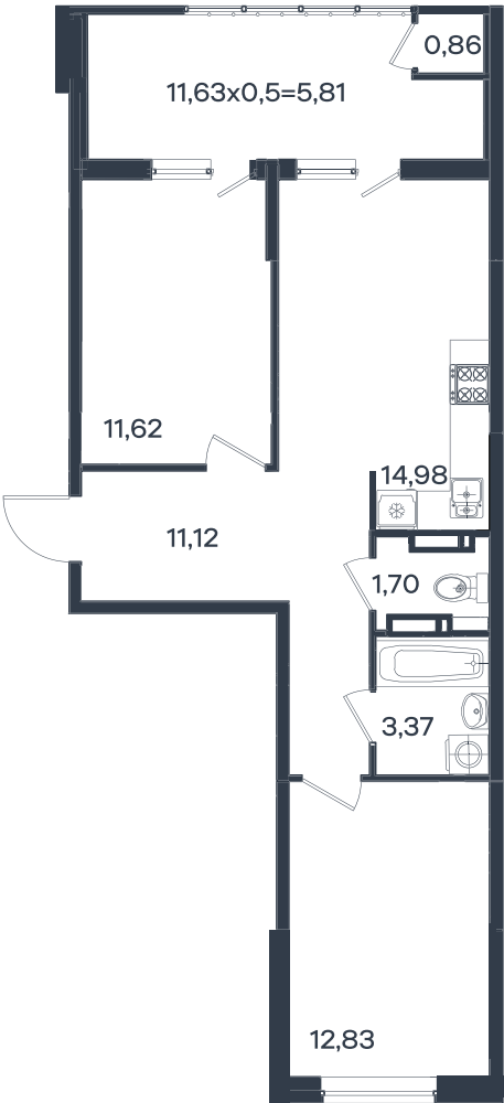
1 этаж
