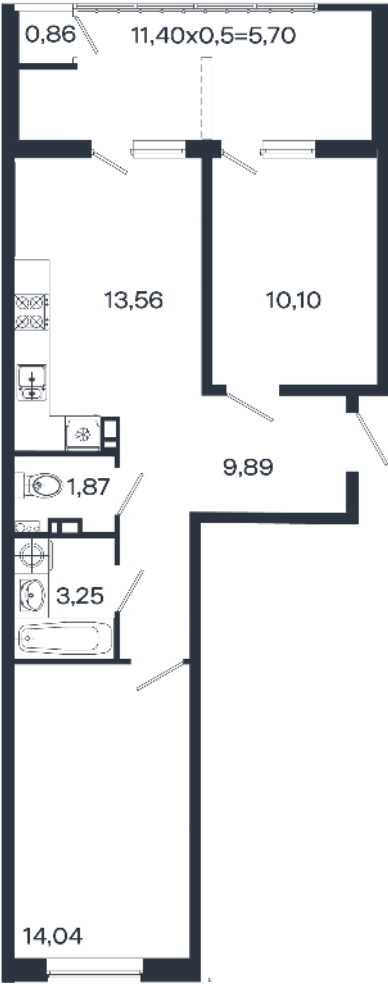
1 этаж
