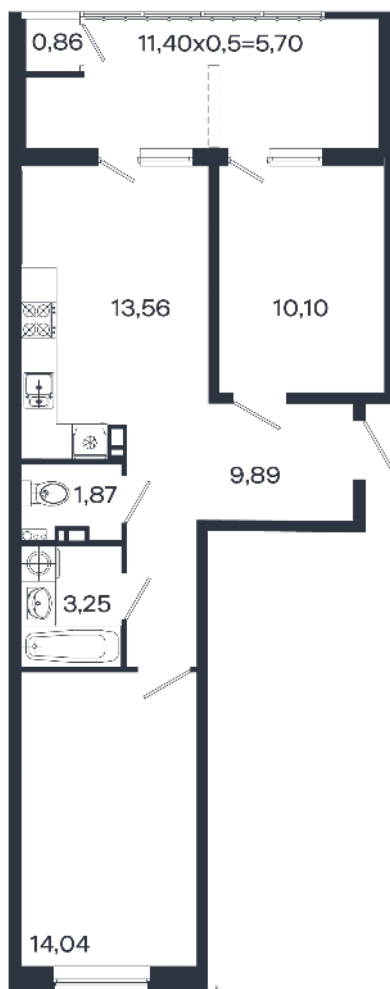
2 этаж
