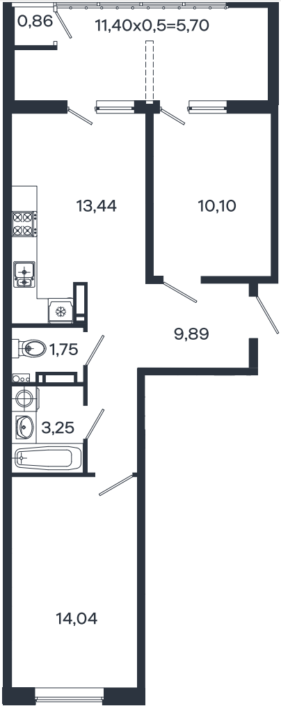
1 этаж
